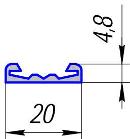
HP-389; 0,124кг/п.м. (ПА-145)
