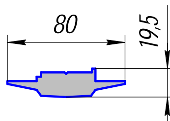
HP-360; 0,901кг/п.м.
