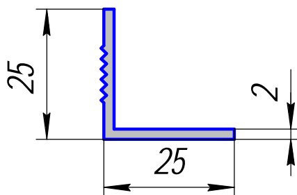
HP-402; 0,261кг/п.м.
