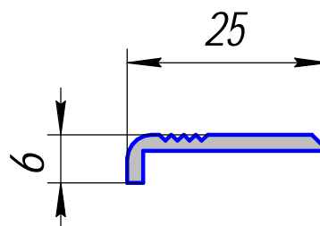
HP-369; 0,140кг/п.м.
