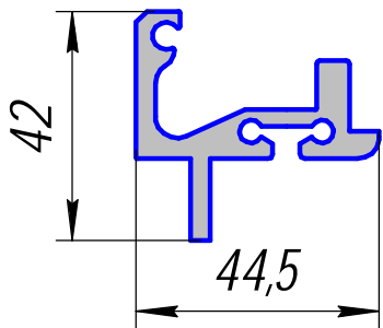
HP-381; 1,201кг/п.м. (ПА-2-10)
