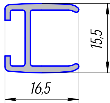
ПО-125-1; 0,178кг/п.м.
