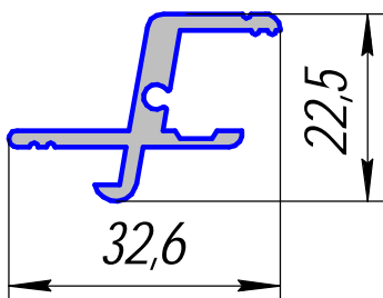
ПА-57; 0,376кг/п.м.
