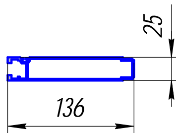
ПА-113; 1,703кг/п.м.
