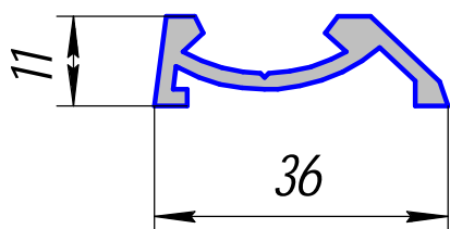
HP-366; 0,356кг/п.м.
