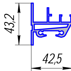
ПА-202; 1,047кг/п.м.
