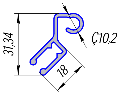
HP-597; 0,421кг/п.м.
