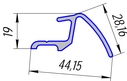
HP-399; 0,453кг/п.м.
