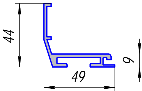
HP-380; 0,758кг/п.м. (ПА-10-10)
