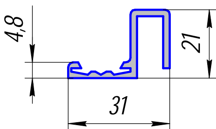
HP-364; 0,366кг/п.м.
