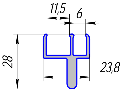
HP-270; 0,430кг/п.м. (ПС 885-1299)
