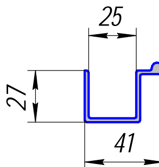
ЭПО-066; 0,547кг/п.м.
