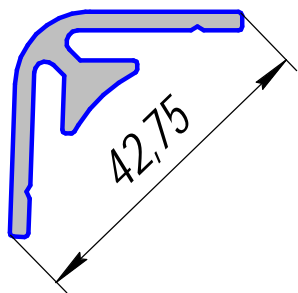
ПА-54; 0,539кг/п.м.
