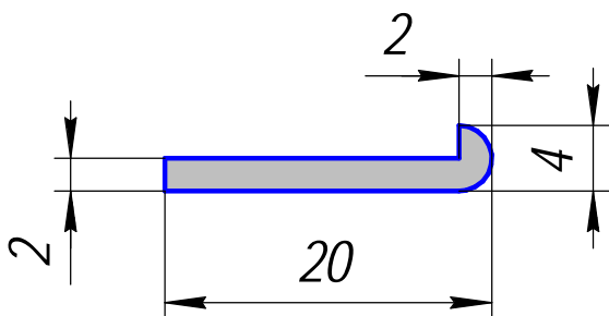
HP-424; 0,115кг/п.м.
