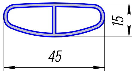
ПА-98; 0,453кг/п.м.
