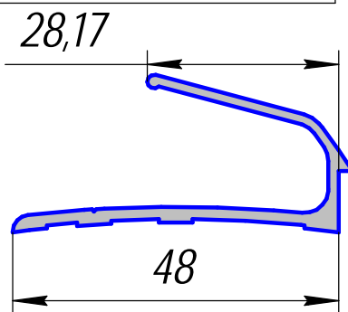
HP-601; 0,749кг/п.м.
