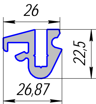
HP-382; 0,654кг/п.м. (ПА-3)
