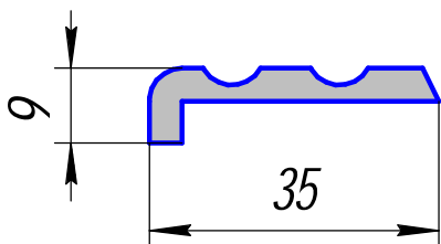
HP-390; 0,360кг/п.м. (ПА-019)
