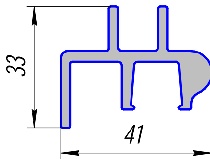
HP-590; 0,926кг/п.м.
