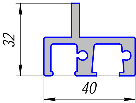
ПА-70; 1,002кг/п.м.
