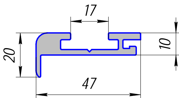
HP-509; 0,757кг/п.м.
