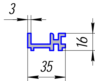
HP-367; 0,663кг/п.м. (ПА-186)
