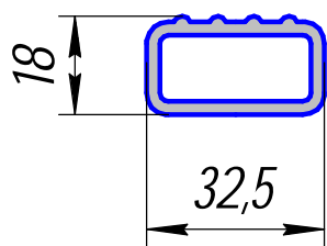
HP-570; 0,595кг/п.м.
