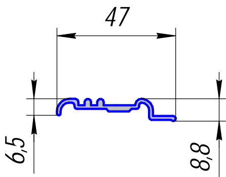
HP-324; 0,295кг/п.м.
