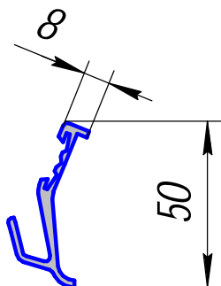
HP-364; 0,366кг/п.м.
