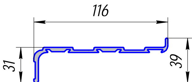
HP-333; 1,156кг/п.м.
