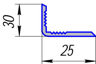
HP-372; 0,177кг/п.м.
