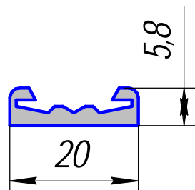
HP-363; 0,179кг/п.м.
