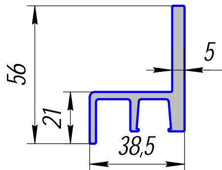
HP-593; 1,227кг/п.м.
