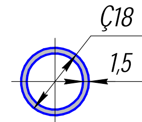
ПА-13; 0,389кг/п.м.
