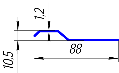
HP-505; 0,303кг/п.м.
