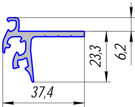
НП-640; 0,52кг/п.м.
