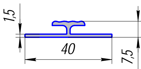
ПА-63; 0,256кг/п.м.
