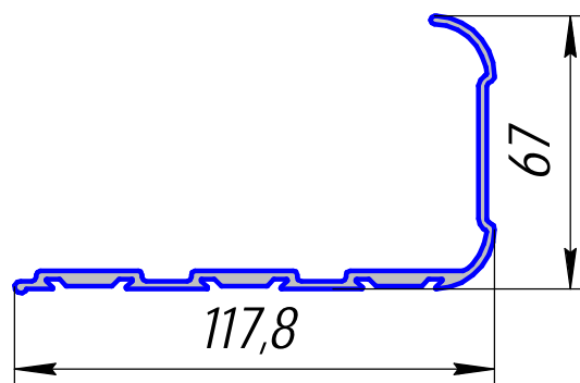
HP-334; 1,339кг/п.м.
