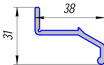
HP-600; 0,420кг/п.м.
