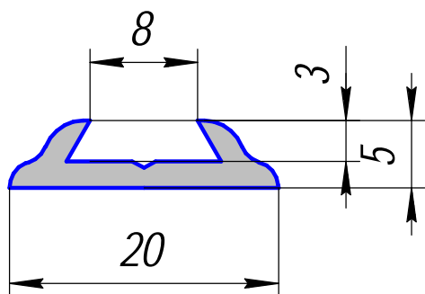
HP-431; 0,137кг/п.м.
