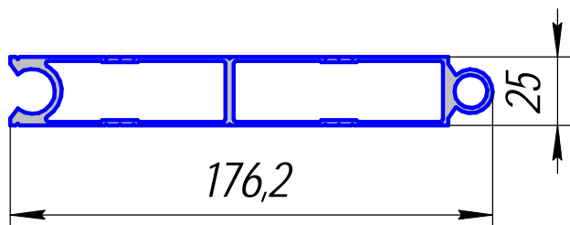
ЭПЗ-026; 2,250кг/п.м.
