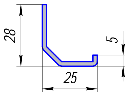
HP-595; 0,266кг/п.м.
