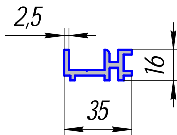
HP-367-01; 0,586кг/п.м. (ПА-186-01)
