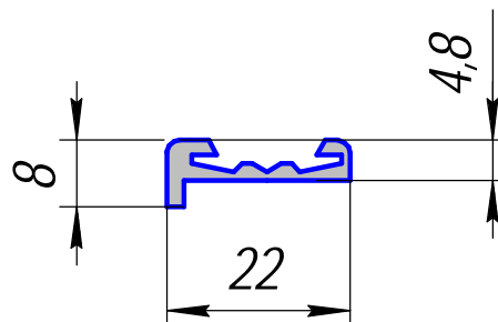
HP-387; 0,869кг/п.м. (ПА-003-01)
