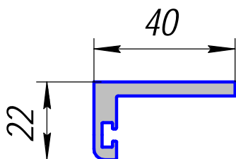
HP-382; 0,654кг/п.м. (ПА-3)
