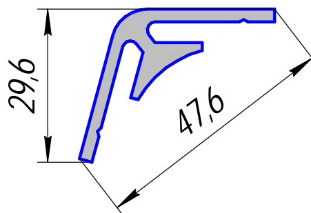
ПА-53; 0,595кг/п.м.
