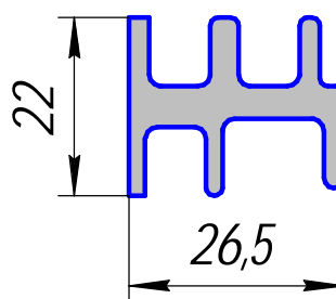
ПА-51; 0,669кг/п.м.
