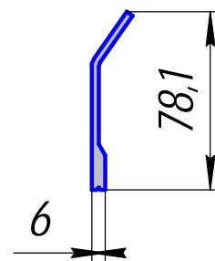
ПА-257; 0,806кг/п.м.
