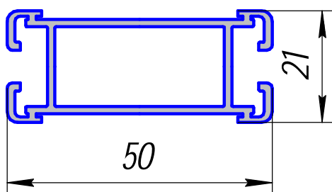
ПА-305; 0,631кг/п.м.
