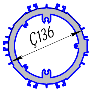
ПА-125; 14,574кг/п.м.
