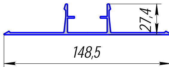
ПА-212; 1,079кг/п.м.
