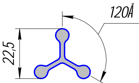
НП-478; 0,361кг/п.м.
