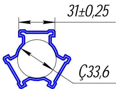
ПА-214; 0,94кг/п.м.
