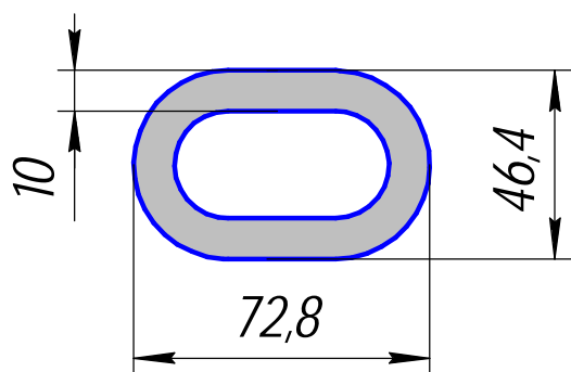
ПА-131; 4,530кг/п.м.
