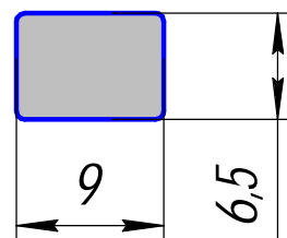
НП-638; 0,295кг/п.м.
