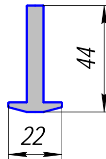
ПА-258; 0,956кг/п.м.
