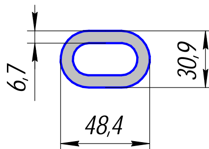
ПА-118; 2,016кг/п.м.
