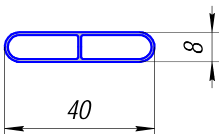
ПА-23; 0,202кг/п.м.
