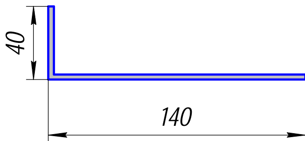
ПА-17; 1,328кг/п.м.
