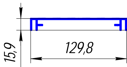
ПА-191-01; 0,709кг/п.м.
