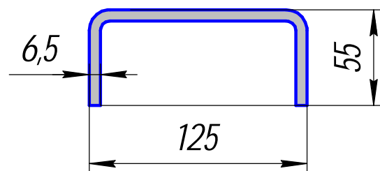
440412; 3,778кг/п.м.
