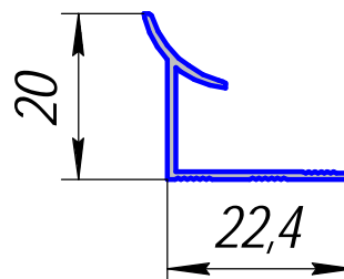
ПА-258; 0,956кг/п.м.
