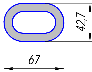
ПА-200; 3,836кг/п.м.
