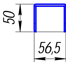
ПА-99; 1,337кг/п.м.
