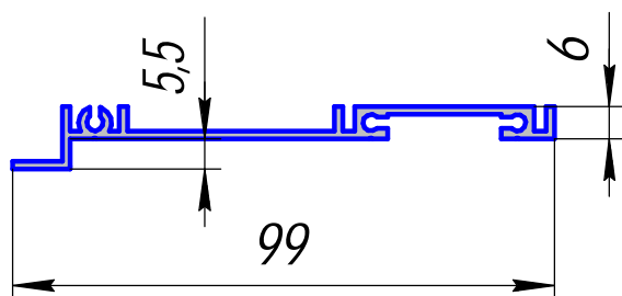
ПА-309; 0,622кг/п.м.
