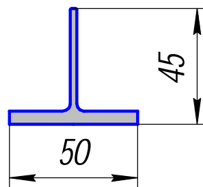
420366; 0,970кг/п.м.
