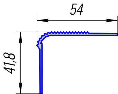
ПА-279; 0,379кг/п.м.
