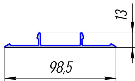
ПА-212; 1,079кг/п.м.
