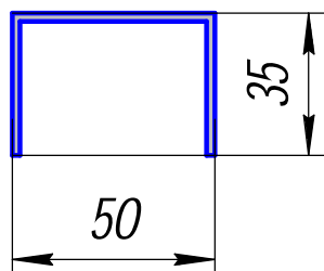
ПА-60; 0,633кг/п.м.
