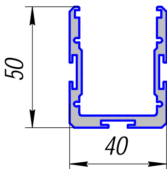
НП-440; 1,244кг/п.м.
