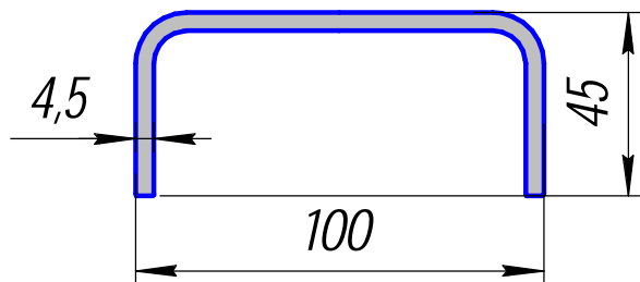
440361; 2,099кг/п.м.
