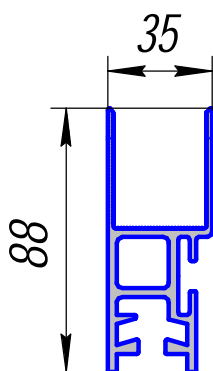
ПА-251; 1,897кг/п.м.
