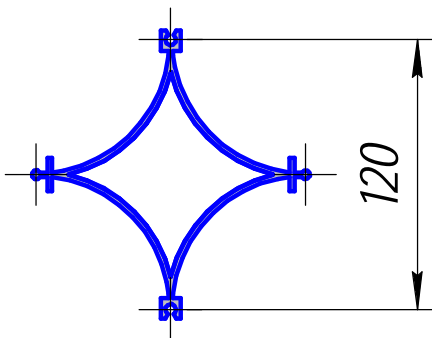
ЭПЗ-001; 2,610кг/п.м.
