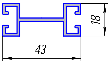
ПА-242; 0,505кг/п.м.
