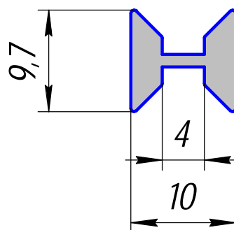
ПА-10; 0,134кг/п.м.
