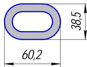
ПА-201; 3,141кг/п.м.
