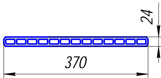
ПА-107; 14,326кг/п.м.
