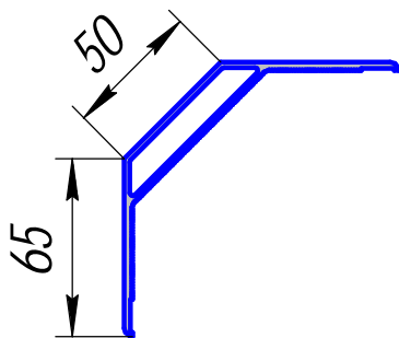
ПА-251; 1,897кг/п.м.
