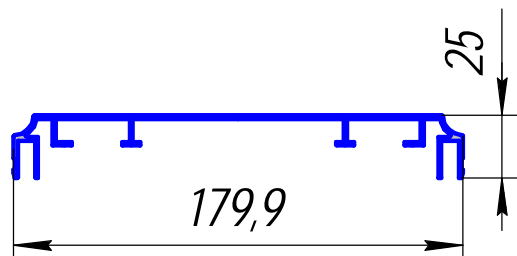
ПА-191-01; 0,709кг/п.м.
