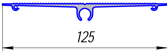
НП-462; 0,840кг/п.м.
