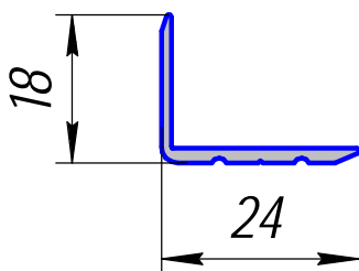
ПА-280; 0,156кг/п.м.
