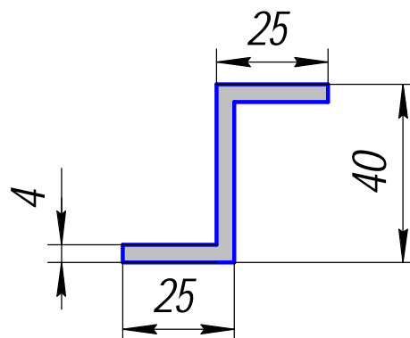
НП-504; 0,889кг/п.м.
