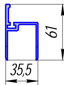
ПА-101; 0,903кг/п.м.
