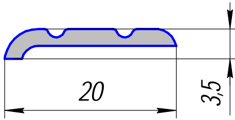
HP-459; 0,097кг/п.м.
