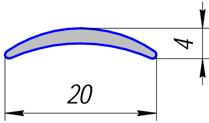
HP-415; 0,092кг/п.м.
