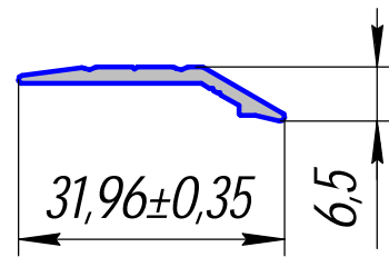
ПА-290; 0,159кг/п.м.
