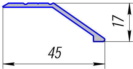
HP-487; 0,246кг/п.м.
