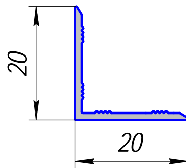
HP-493; 0,129кг/п.м.
