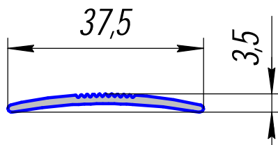
HP-464; 0,165кг/п.м.
