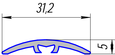
HP-415; 0,092кг/п.м.
