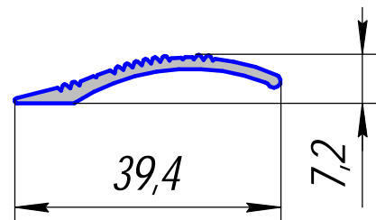
ПА-291; 0,199кг/п.м.
