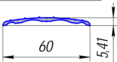
HP-460; 0,176кг/п.м.
