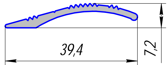
HP-485; 0,222кг/п.м.
