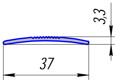
ПА-286; 0,151кг/п.м.
