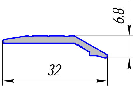
HP-486; 0,182кг/п.м.
