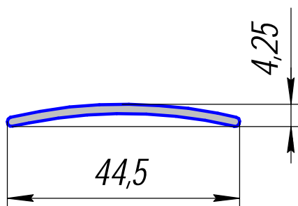
ПА-286; 0,151кг/п.м.
