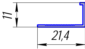
HP-451; 0,085кг/п.м.
