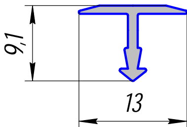
HP-446; 0,063кг/п.м.
