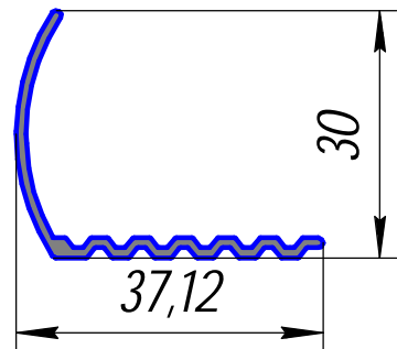
HP-491; 0,231кг/п.м.
