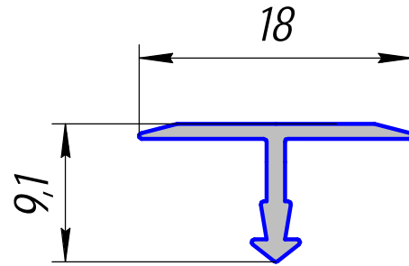
HP-447; 0,135кг/п.м.
