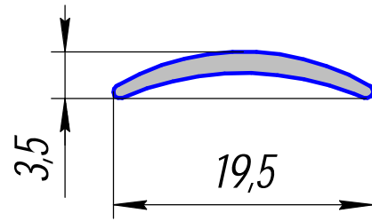
ПА-288; 0,075кг/п.м.
