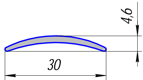
HP-455-01; 0,106кг/п.м.
