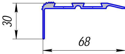
НП-495; 0,519кг/п.м.
