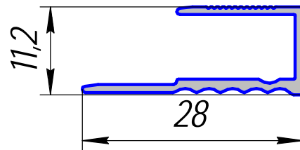
HP-450; 0,154кг/п.м.
