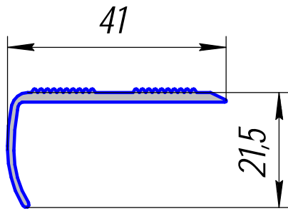
НП-494; 0,279кг/п.м.
