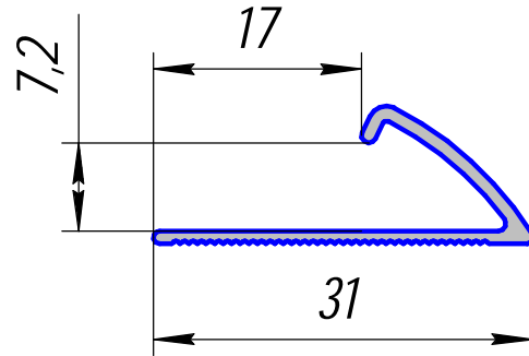
HP-465; 0,135кг/п.м.
