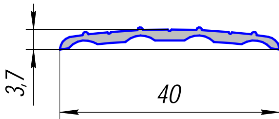
HP-459; 0,097кг/п.м.
