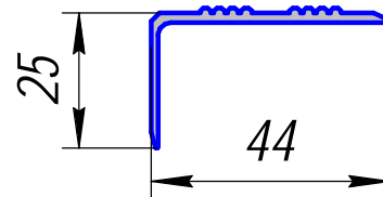
HP-483; 0,318кг/п.м.
