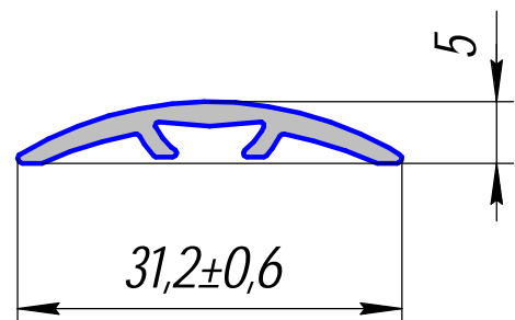
ПА-295; 0,166кг/п.м.
