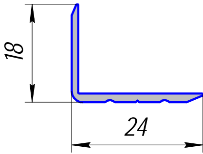
HP-458; 0,145кг/п.м.
