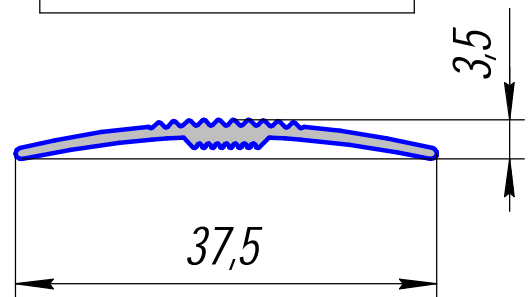
HP-456; 0,142кг/п.м.
