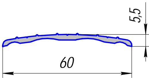
HP-416; 0,178кг/п.м.
