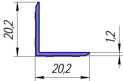
HP-492; 0,128кг/п.м.
