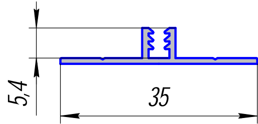
HP-447; 0,135кг/п.м.
