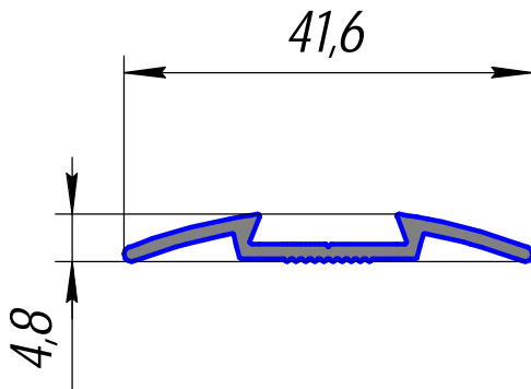
HP-488; 0,203кг/п.м.
