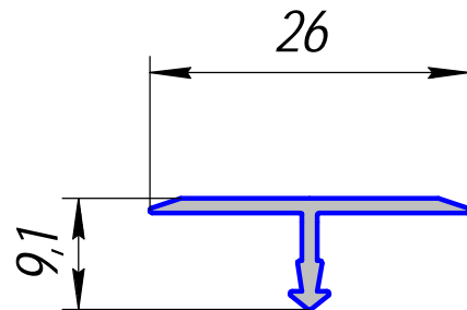
HP-448; 0,077кг/п.м.
