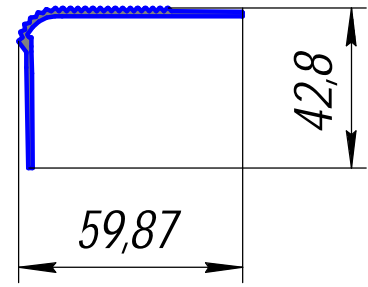
HP-490; 0,428кг/п.м.
