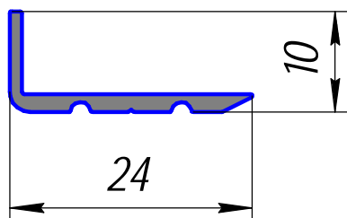
HP-489; 0,127кг/п.м.
