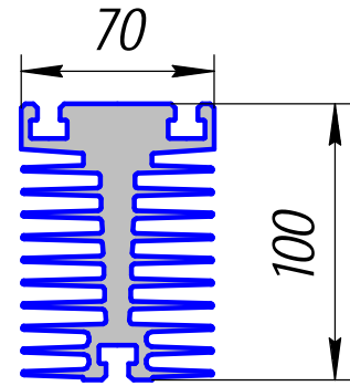
ПА-229; 8,525кг/п.м.
