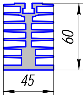
ПА-195; 3,048кг/п.м.
