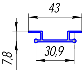
HP-272; 0,274кг/п.м.
