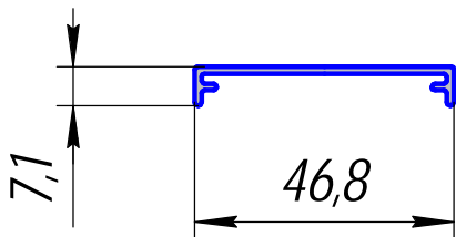
HP-273; 0,222кг/п.м.
