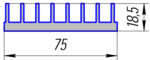
ПА-229; 8,525кг/п.м.
