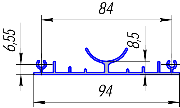
HP-271; 0,647кг/п.м.
