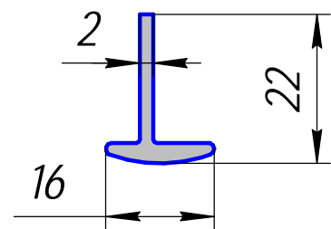
АПР 290; 0,211кг/п.м.
