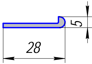
АПР 291-1; 0,169кг/п.м.
