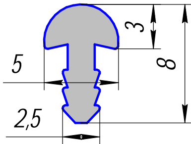
АС-69; 0,059кг/п.м.
