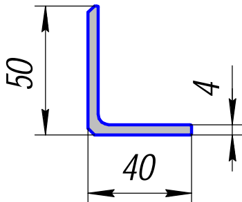
АУ-84; 0,924кг/п.м.
