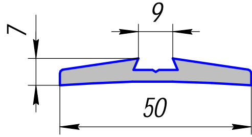
ПК 02090-2; 0,606кг/п.м.
