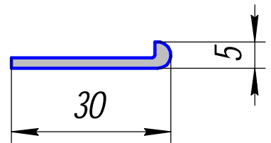
АПР 254; 0,180кг/п.м.
