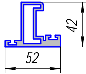
АС-76; 1,460кг/п.м.
