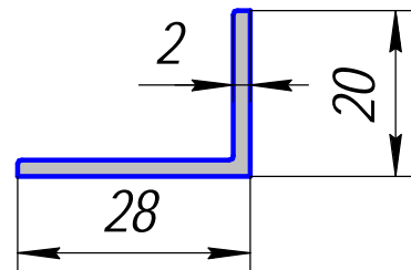
ПК 8271; 0,249кг/п.м.
