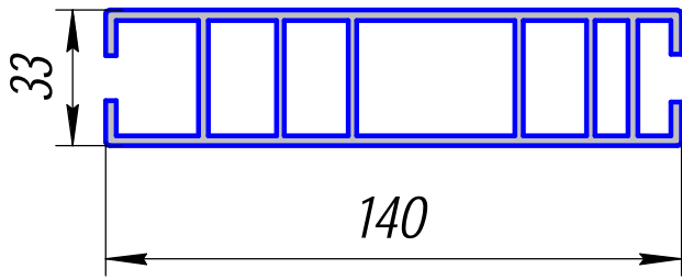
ПК 02090-6; 3,108кг/п.м.
