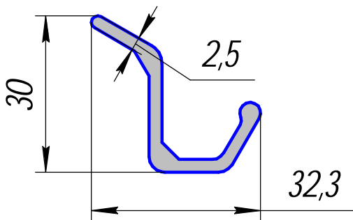
ПК 02105; 0,442кг/п.м.
