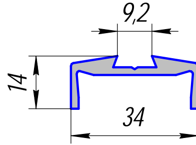
ПК 8268; 0,795кг/п.м.
