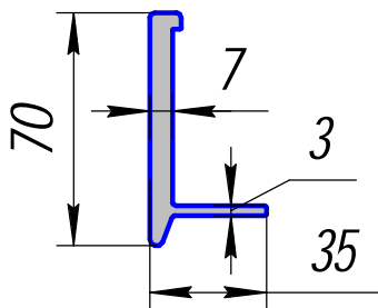
АС-59; 1,540кг/п.м.
