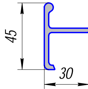
АПР-277; 0,649кг/п.м.
