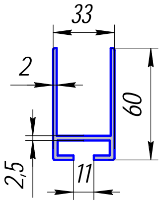
АС-68; 0,988кг/п.м.
