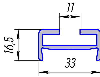
ПК 02090-3; 0,433кг/п.м.
