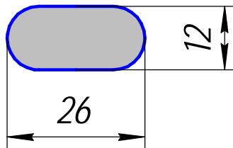
ПК 805-4; 0,762кг/п.м.
