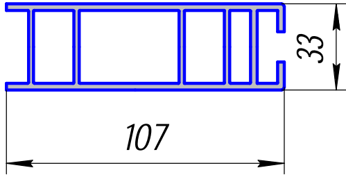
АС-83; 2,358кг/п.м.
