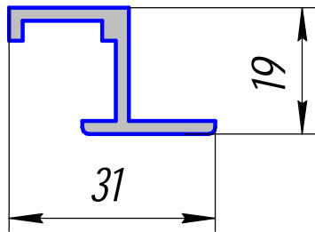
ПК 02082; 0,319кг/п.м.
