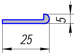
АПР 291-1; 0,169кг/п.м.
