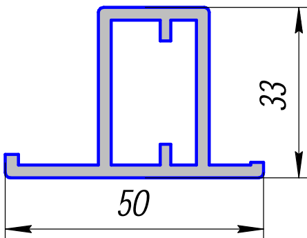
АС-73; 0,922кг/п.м.
