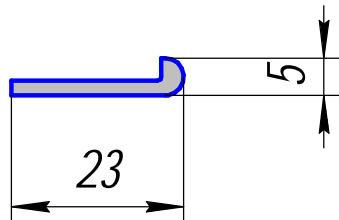
АПР 143; 0,142кг/п.м.
