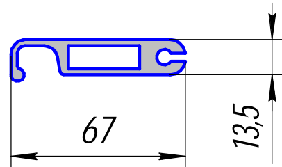
АС-63; 1,191кг/п.м.
