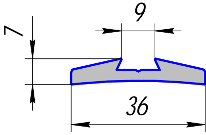
ПВ-1182; 0,424кг/п.м.
