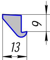
АПР 120; 0,217кг/п.м.
