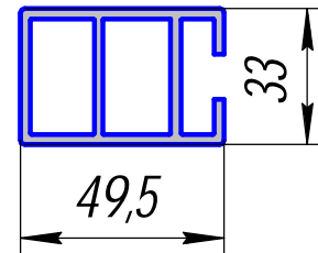
АС-78; 1,315кг/п.м.
