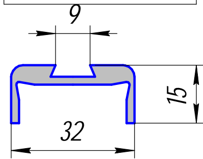
ПК 02090-3; 0,433кг/п.м.
