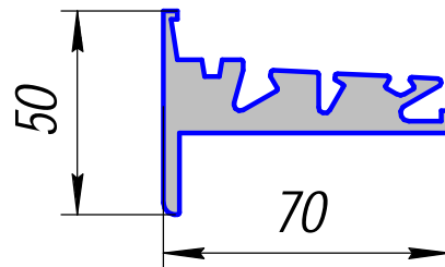
НП-266; 2,624кг/п.м.
