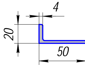
ПК 111-17; 0,591кг/п.м.
