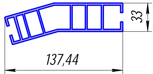
АС-79; 3,047кг/п.м.
