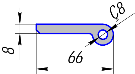
АС-85; 1,633кг/п.м.
