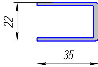
АС-64; 0,478кг/п.м.
