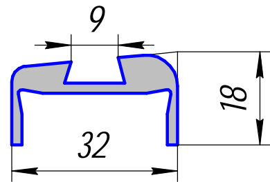
ПК 02090-5; 0,499кг/п.м.
