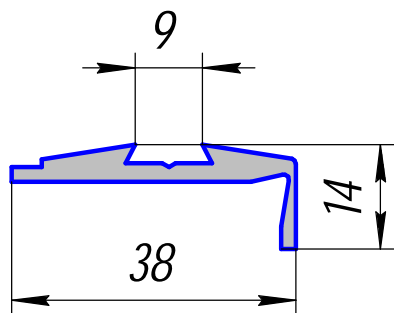
ПК 8267; 0,377кг/п.м.
