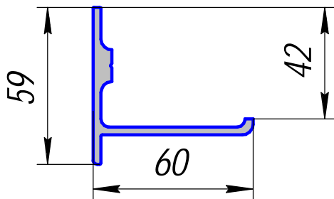
КП-2042; 1,115кг/п.м.
