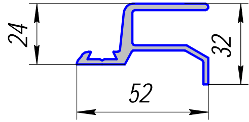
ПК 8268; 0,795кг/п.м.
