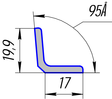
ПВ 1717; 0,292кг/п.м.
