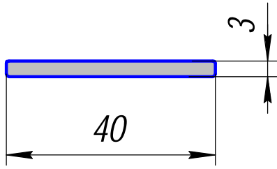
ПК 801-3; 0,325кг/п.м.
