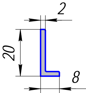
АПР 144; 0,141кг/п.м.
