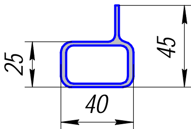
ПК 02090-8; 0,858кг/п.м.
