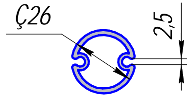
АС-62; 0,469кг/п.м.
