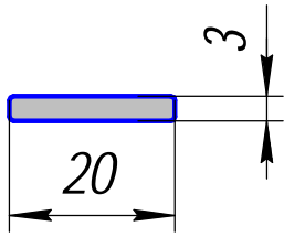
ПК 801-144; 0,162кг/п.м.
