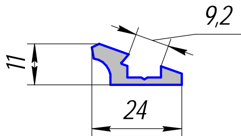
ПК 8271; 0,249кг/п.м.
