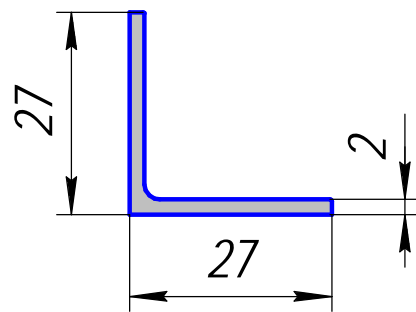
НП-637; 0,284кг/п.м.
