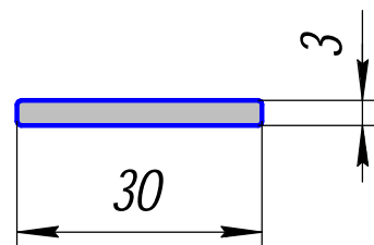
ПК 801-2; 0,243кг/п.м.
