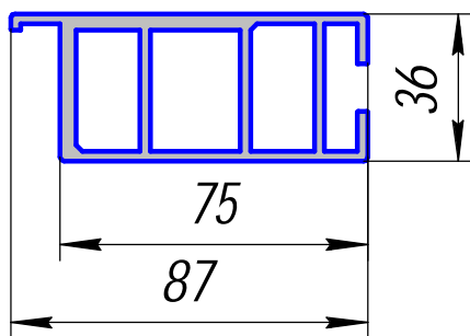
АС-75; 2,362кг/п.м.
